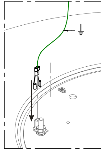
DETTAGLIO A
