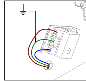
DETTAGLIO A
