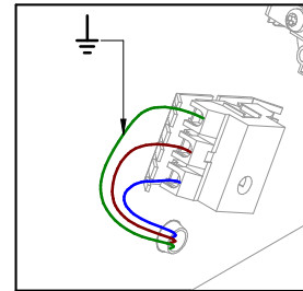
DETTAGLIO A 1:2.5
